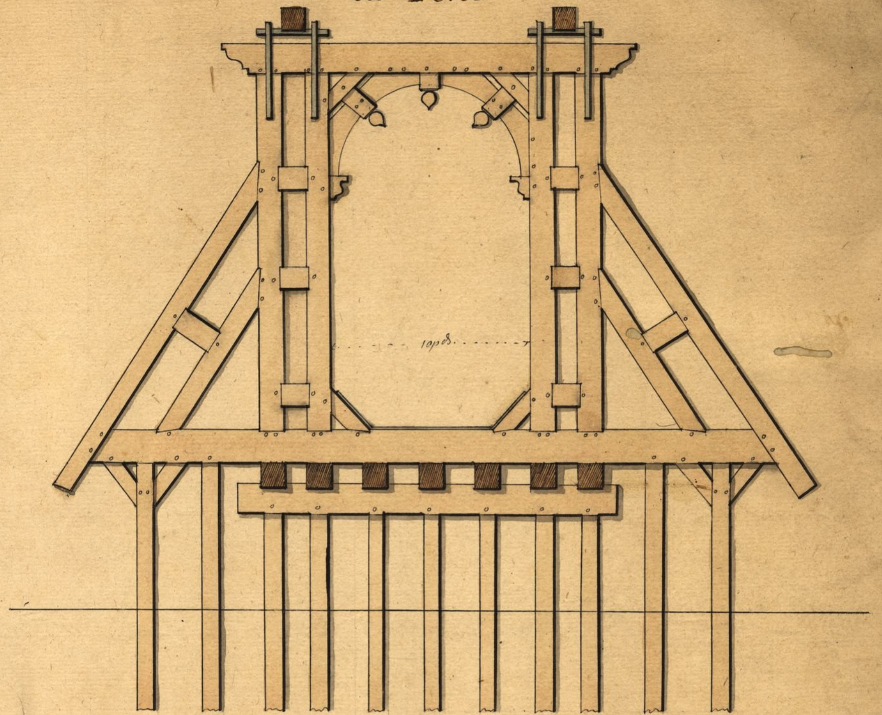
Elevation de la Porte du Pont
